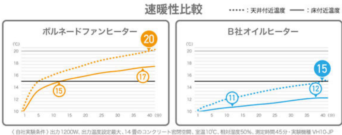
速暖性比較グラフ
