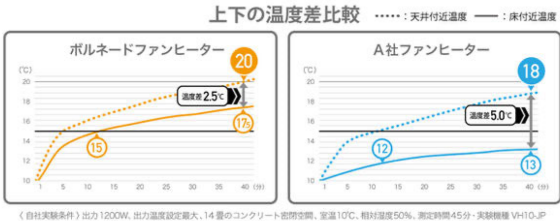
上下の温度差グラフ
